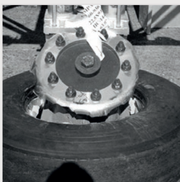
Roată din aluminiu turnat
